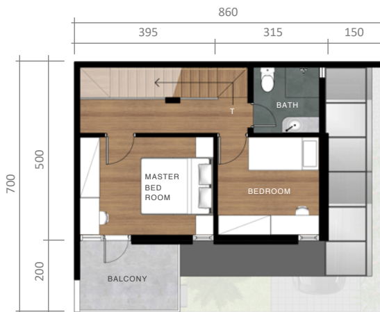
LANTAI 2
